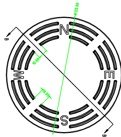
612系列太陽能警示埋地燈細部圖
