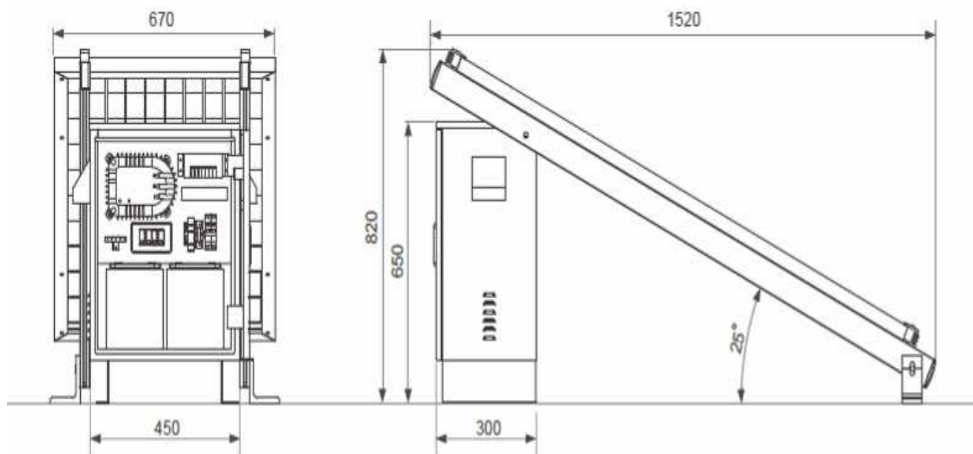
太陽能獨立型套件系列 ST-130 規範圖
