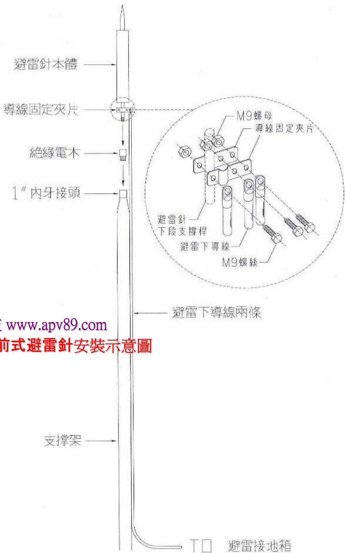
避雷針組裝示意圖
